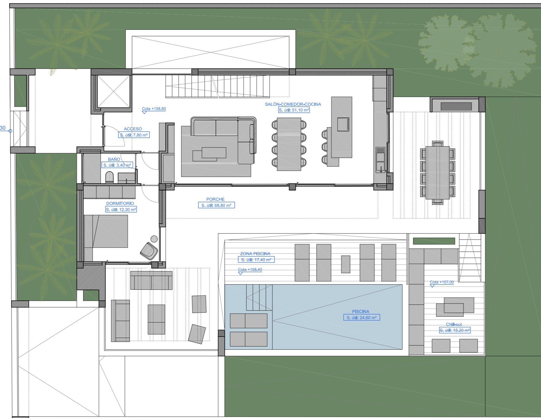
PLANTA BAJA DE VIVIENDA. Sup. Construida: 88,90 m 2 + 86,20 m 2 de porche
