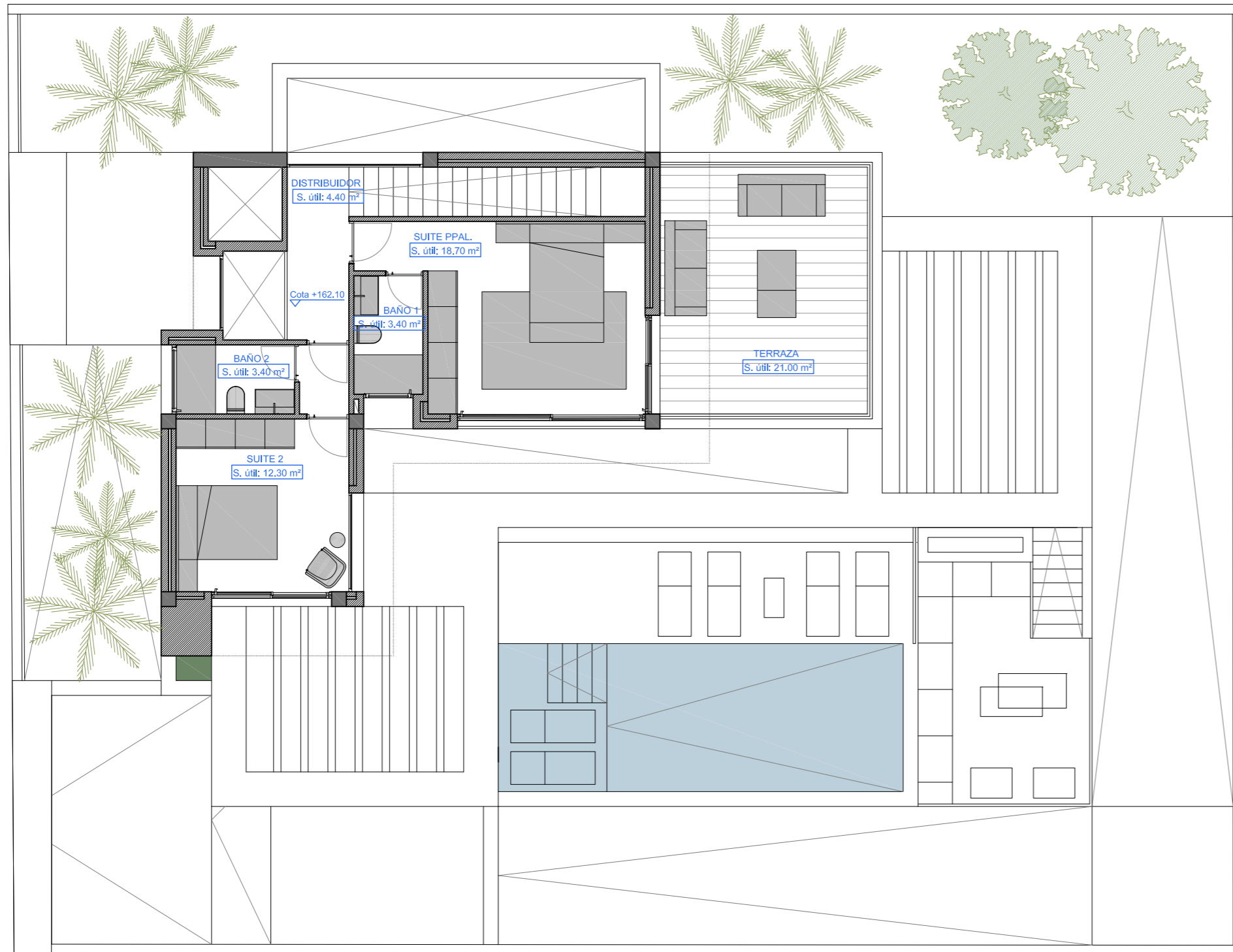
PLANTA ALTA DE VIVIENDA. Sup. Construida: 55,40 m 2 + 21,00 m 2 de terraza
