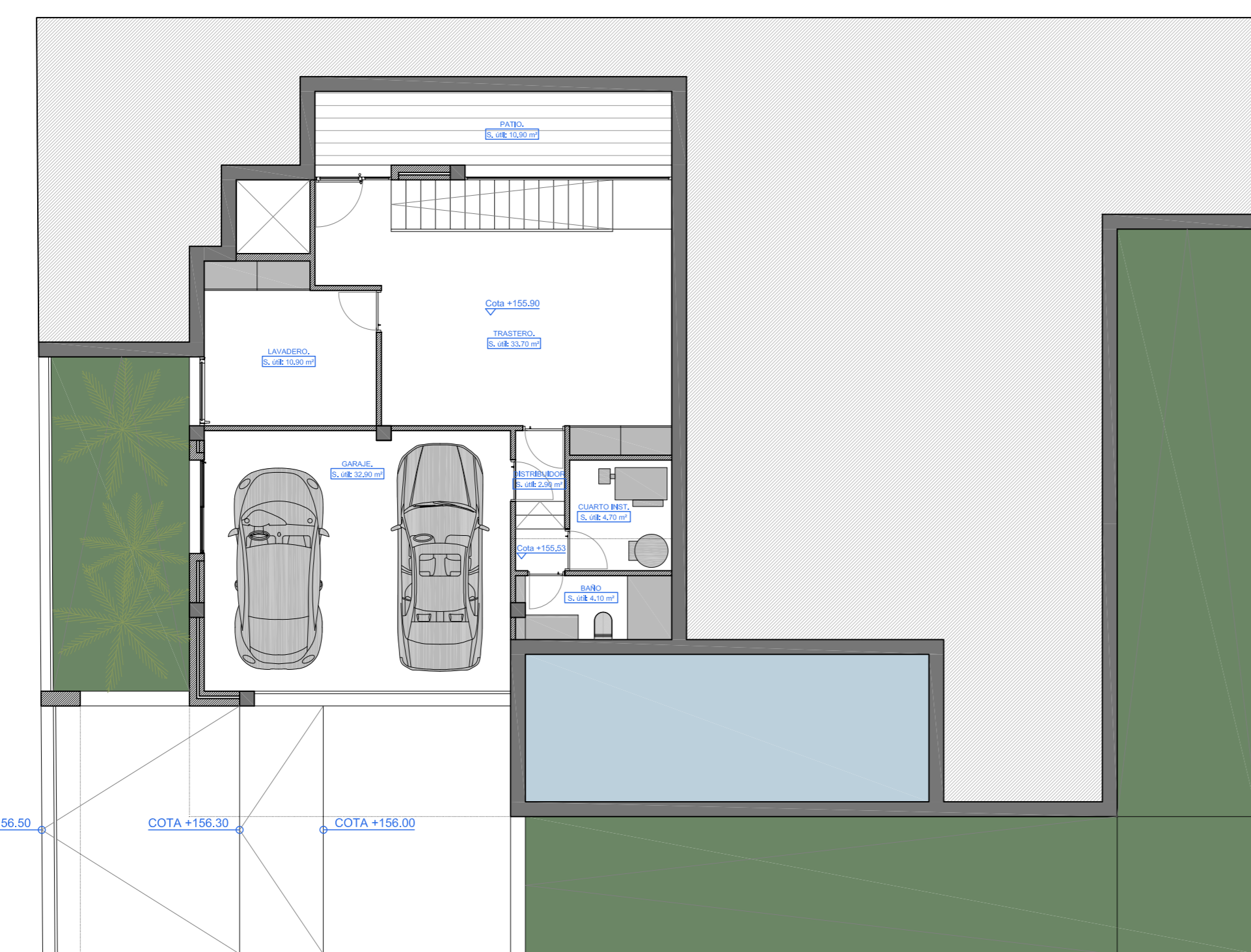
PLANTA SÓTANO DE VIVIENDA. Sup. Construida: 106,60 m 2
